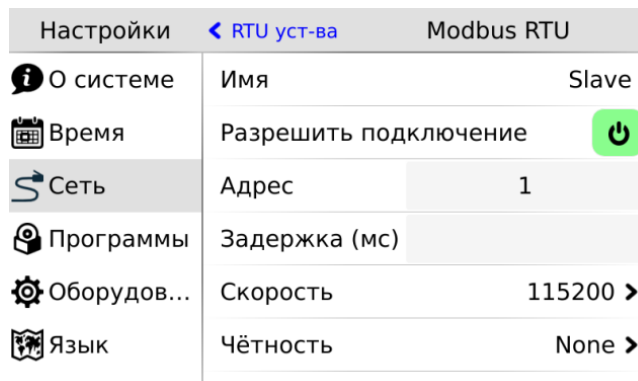
Рис. 31 – Настройки Modbus RTU slave.
