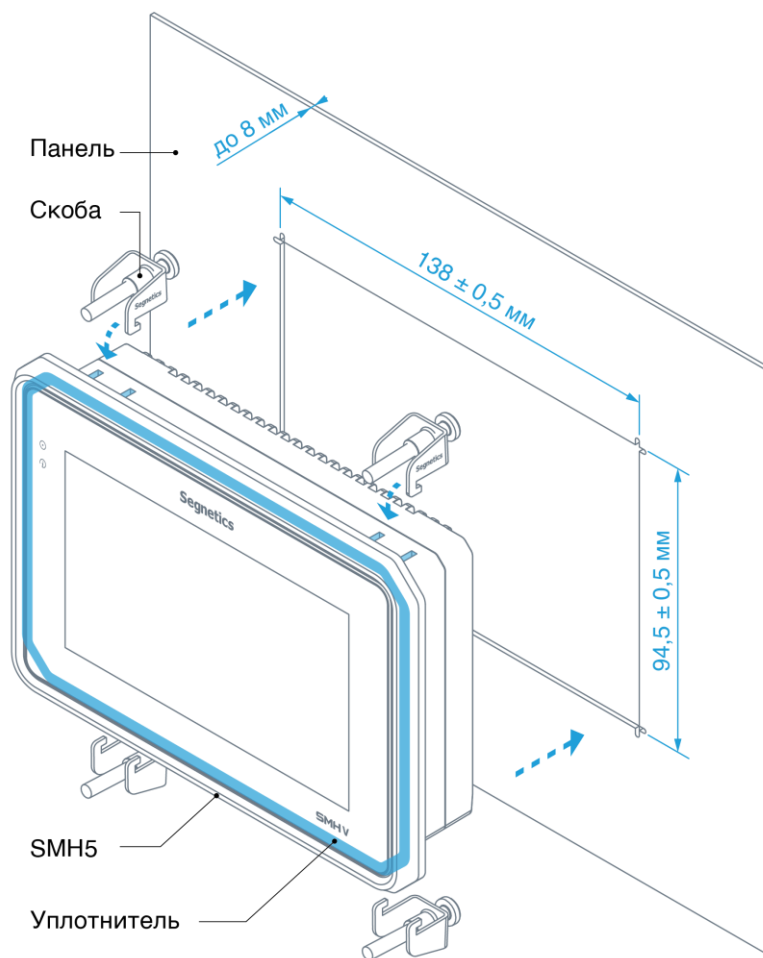
Рис. 58 - Монтаж контроллера.
